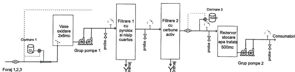
Schema de tratare apa Draganesti- Neamt
